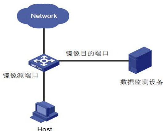
图 4-1 镜像示意图
