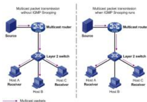
图 4-2 IGMP 对比图
